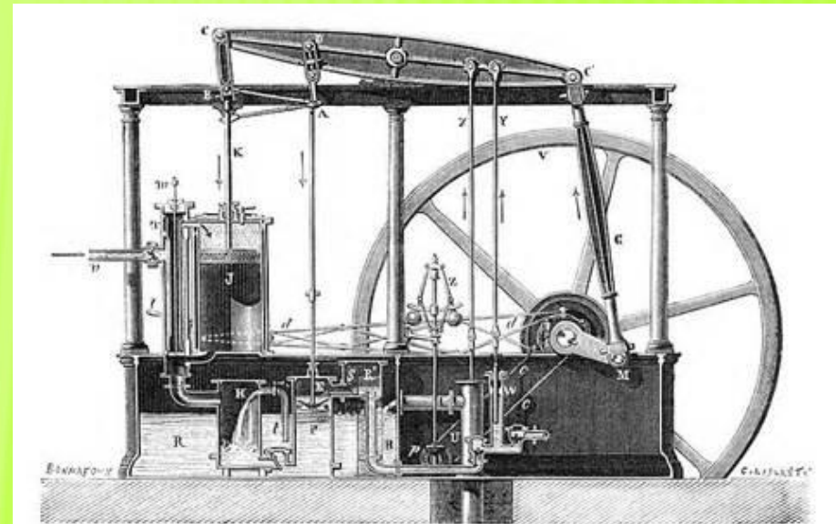
Fig. 59. — Machine à balancier de Watt.
